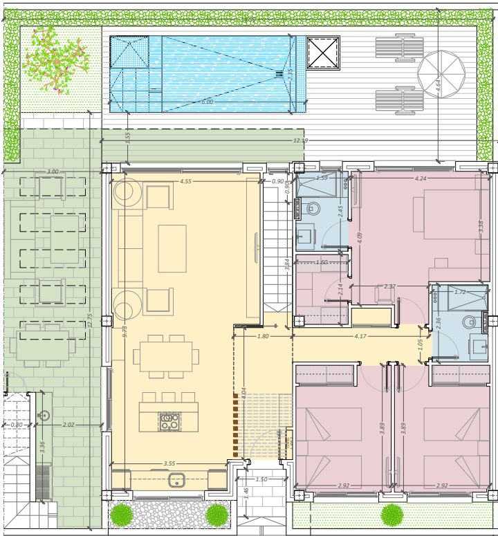
PLANTA BAJA
