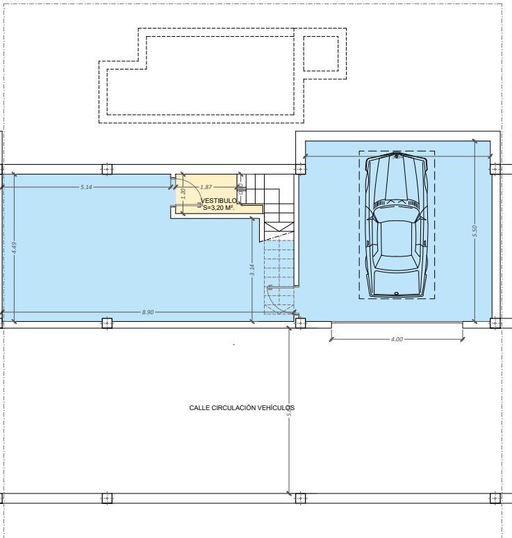
PLANTA SOTANO
